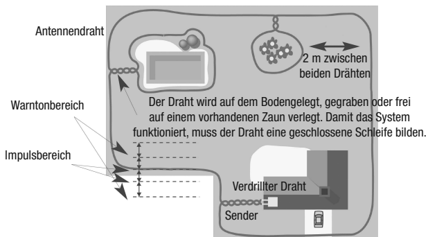
Abb. 3 – Installationsbeispiel
