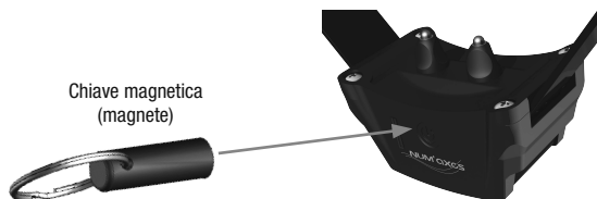
Fig. 5 Accensione e spegnimento del collare ricevitore con la chiave magnetica
