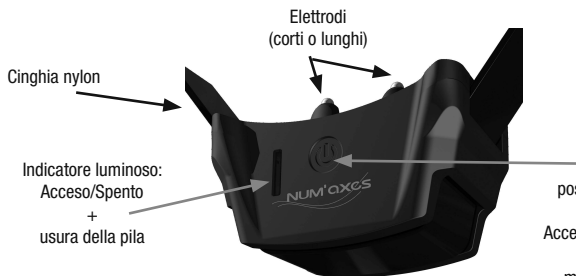
Fig. 2 - Collare ricevitore
