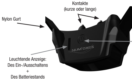
Abb. 3 - Empfänger-Halsband
