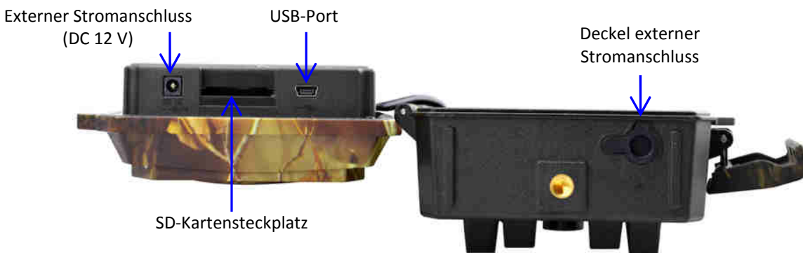
Bild 3: Innenansicht
