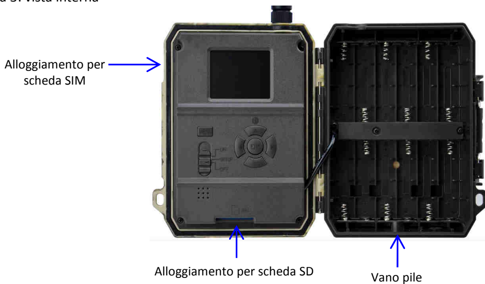
Figura 3: vista interna
