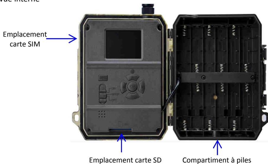
Figure 3 : vue interne
